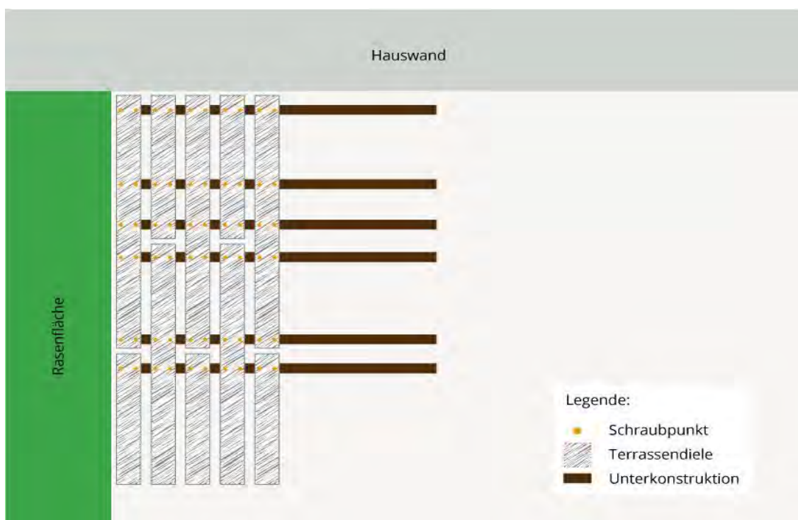
Verlegung mit zwei Stößen in der Fläche
