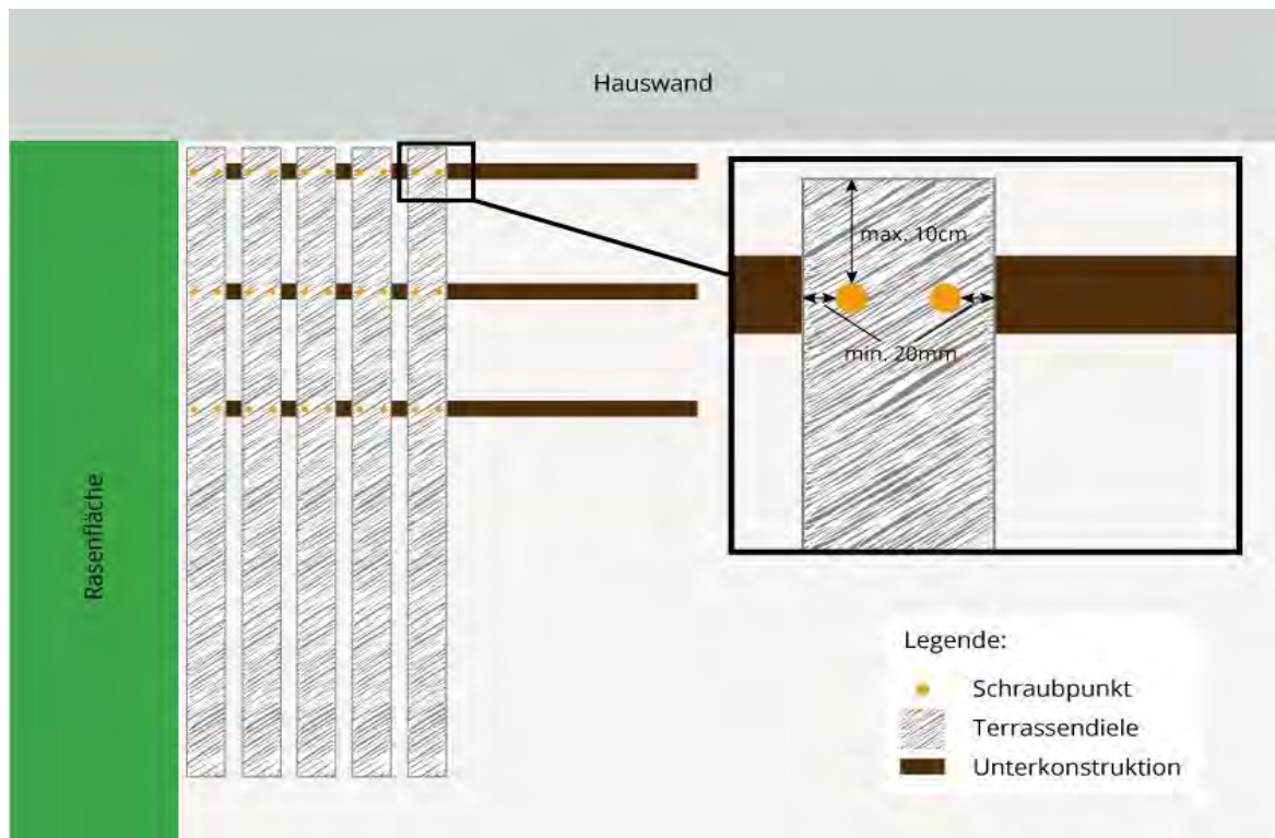
Verlegung über die volle Länge
